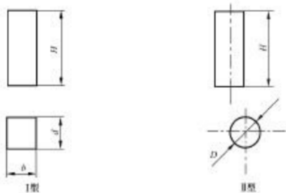
图 1 试样型式
